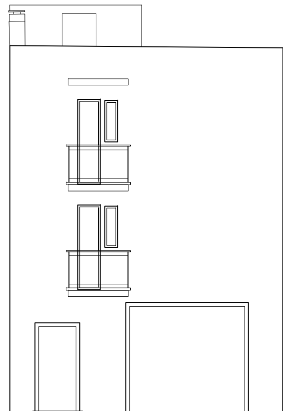
Alzado Acceso Plantas Superiores
